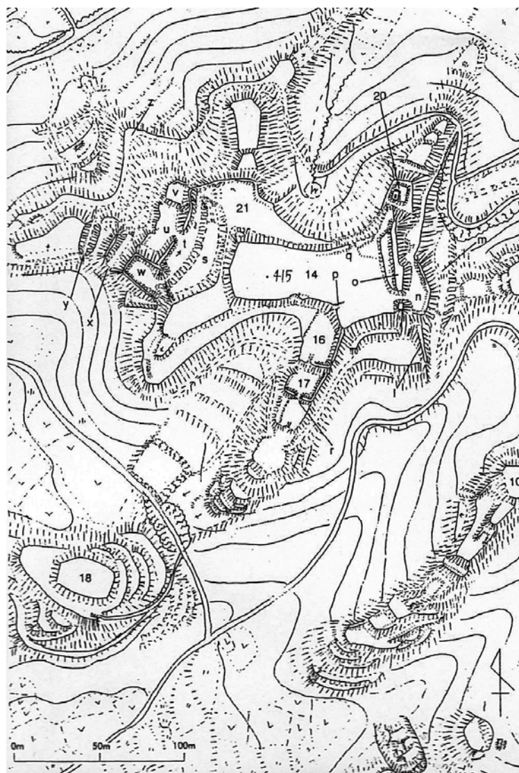
図6 竹貫城主要部詳細図
