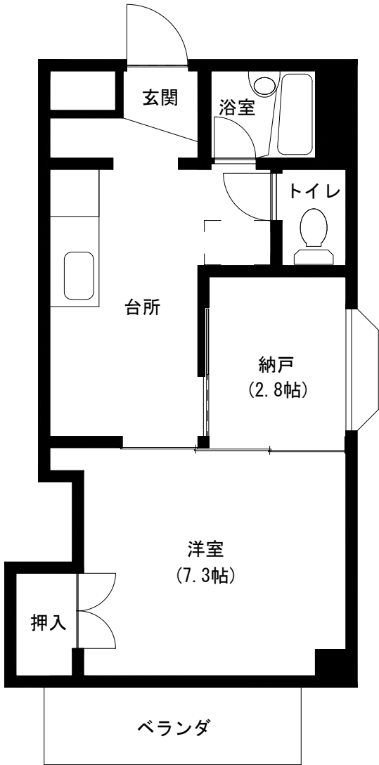
2、3階平面図
